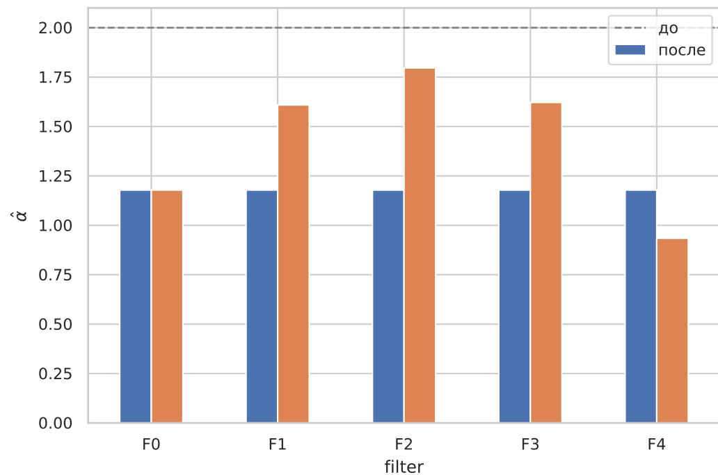
Хвостовой индекс \alpha до / после
