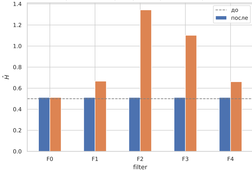
Хёрст до / после фильтрации (среднее по корзине)
