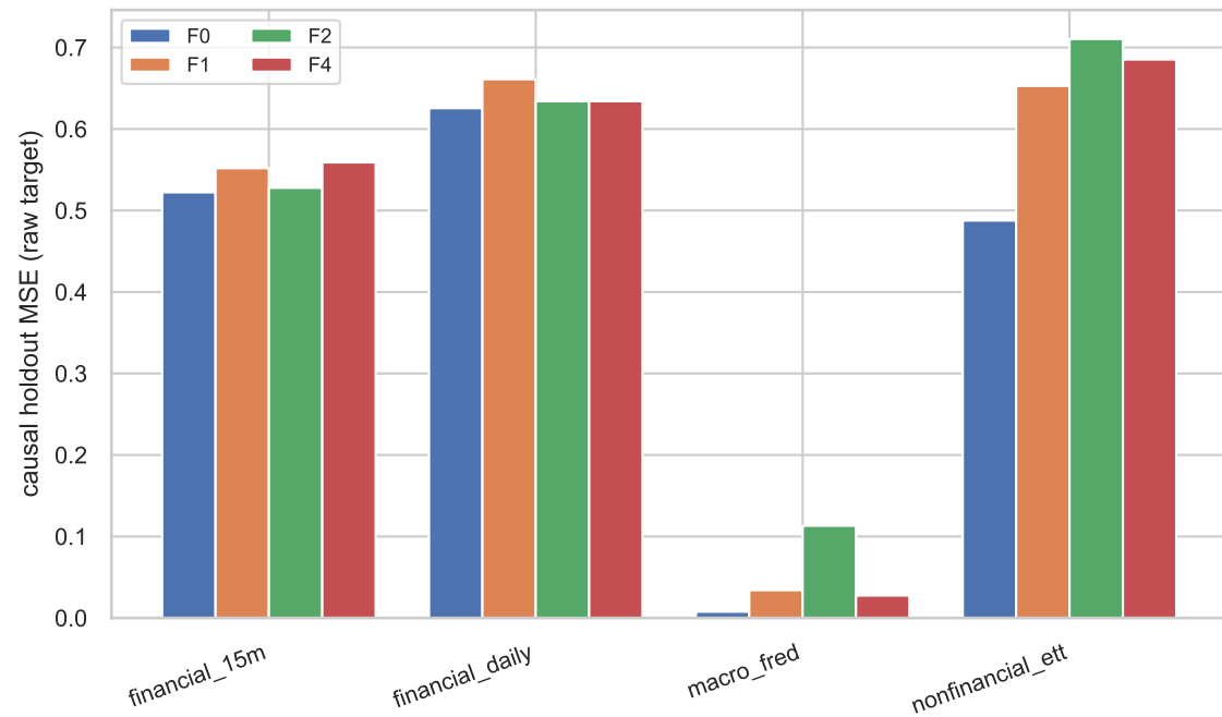
(б) Качество прогноза (causal walk-forward)
