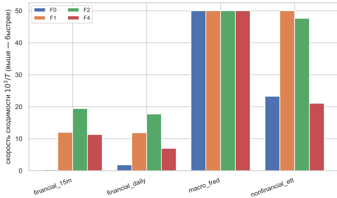
(а) Скорость по доменам; T — итераций до 100 \times падения \|\nabla f\|^2 (Adam)
