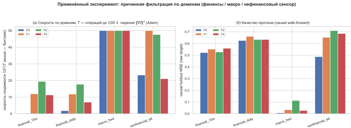
Рис. 3. Применённый causal-эксперимент по доменам (Adam): (а) скорость сходимости 10^3/T ( T — итераций до 100× падения \|\nabla f\|^2 ; выше — быстрее); (б) causal walk-forward holdout MSE. На фин. 15-мин F2 спасает сходимость ( \approx 78\times ) без потери качества.
