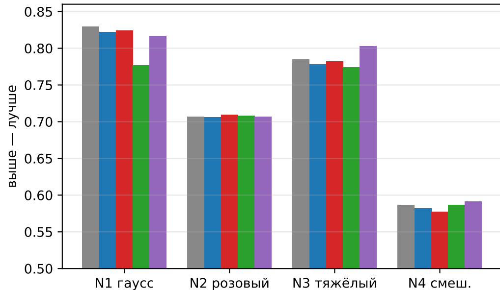
Логистическая: holdout-точность
