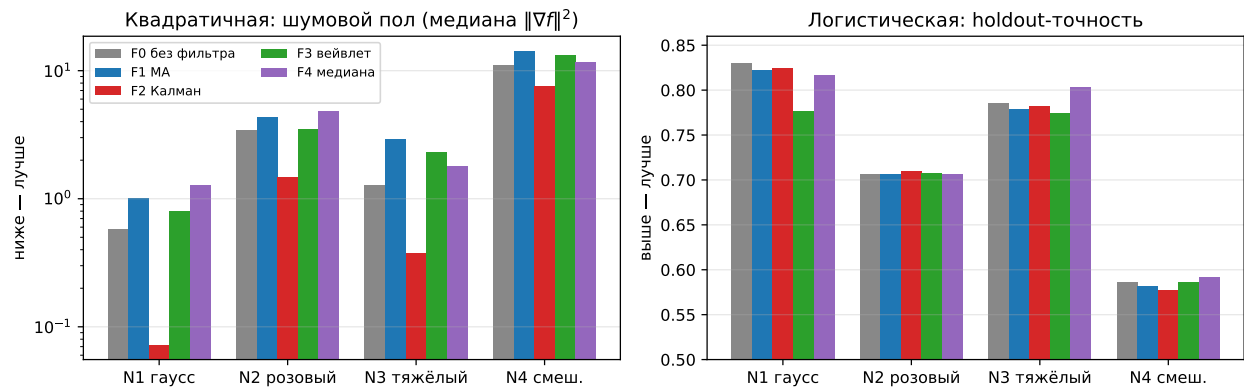
Рис. 3. Синтетический факторный итог. Слева — шумовой пол на квадратичной задаче (лог-шкала, ниже лучше); справа — holdout-точность логистической (выше лучше). Калман доминирует по полу, медиана — по точности на тяжёлых хвостах N3/N4.
