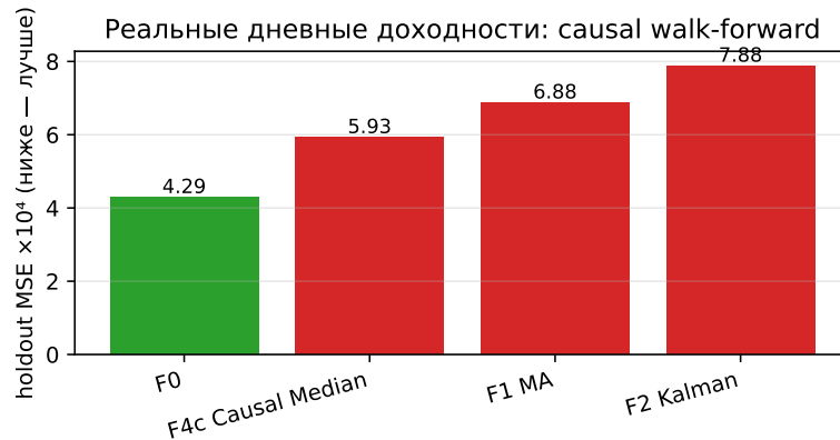
Рис. 4. Реальные дневные доходности, causal walk-forward: holdout MSE по фильтрам. Контроль F0 (зелёный) — лучший; любой causal-фильтр ухудшает прогноз.
