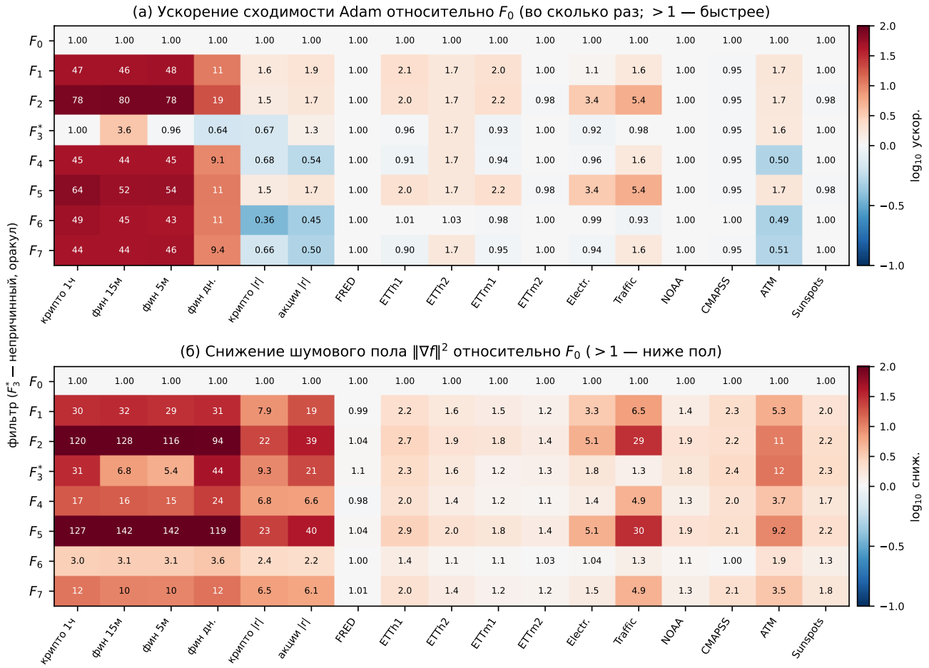
Рис. 2. Полная карта блока D: все фильтры F_0 – F_7 на всех 17 доменах (Adam, регрессия AR(5), 4 сйда). (а) ускорение сходимости относительно F_0 (во сколько раз; > 1 — быстрее); (б) снижение шумового пола \|\nabla f\|^2 относительно F_0 . Выигрыш сосредоточен на тяжёловостовых доходностях (левый блок): линейный Калман F_2 и каскад F_5 дают 44–142×, причём по полу каскад F_5 — лучший; на светлостовых/гладких рядах (FRED, ETT, NOAA, sunspots) все фильтры \approx 1 \times . F_3^* — непричинный оракул, в рекомендованное правило не входит.
