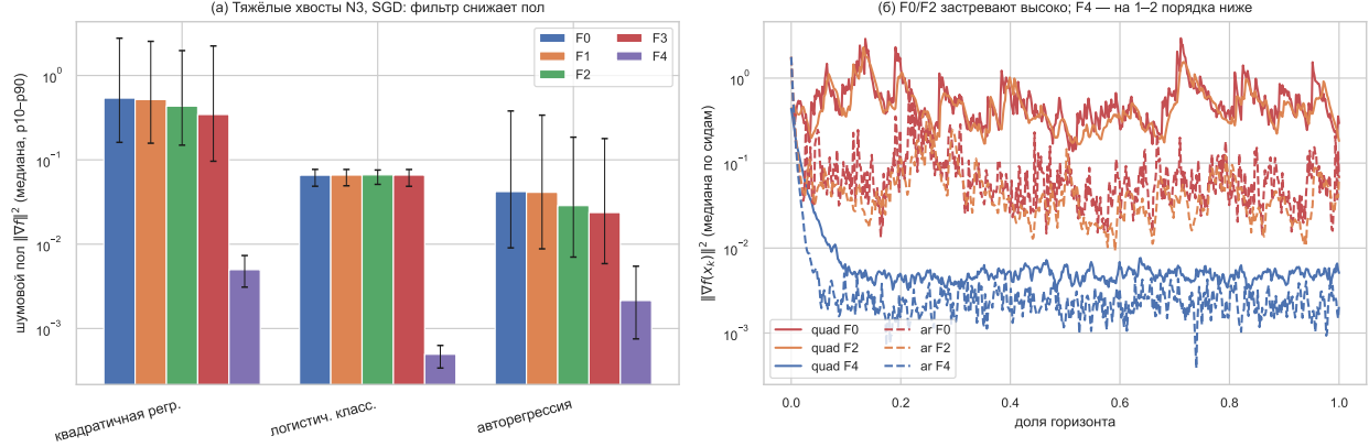
Рис. 1. N_3 , SGD, 8 сидов. (а) пол F_0 – F_4 , лог-шкала, p_{10} – p_{90} ; (б) медиана \|\nabla f\|^2 : F_0/F_2 застревают, F_4 падает на 1–2 порядка. Линейные и вейвлет-фильтры идут вдоль F_0 (Утверждение 1).
