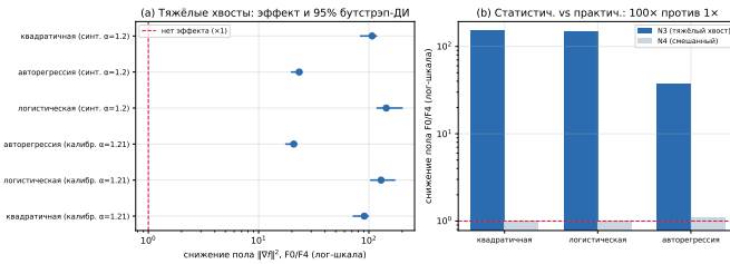
Рис. 5: Слева — лесовидная диаграмма снижения асимптотического уровня F0/F4 при тяжёлых хвостах с 95%-ми бутстрэп-интервалами: для всех задач — и на синтетике ( \alpha = 1.2 ), и на калиброванном под реальные данные шуме ( \alpha = 1.21 ) — интервал целиком правее линии «нет эффекта» ( \times 1 ). Справа — контраст статистической и практической значимости: на N3 фильтр снижает пол в \sim 100 раз, на смешанном N4 — лишь в \sim 1.1 , у самой границы \times 1 (лог-шкала).
