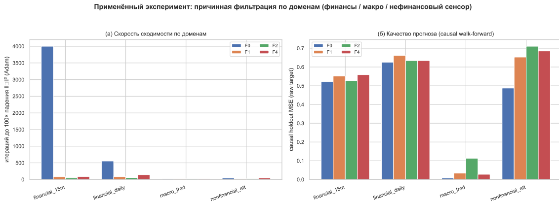
Рис. 3. Применённый causal-эксперимент по доменам (Adam): (а) итераций до сходимости; (б) causal walk-forward holdout MSE. На фин. 15-мин F2 спасает сходимость ( \approx 78\times ) без потери качества.
