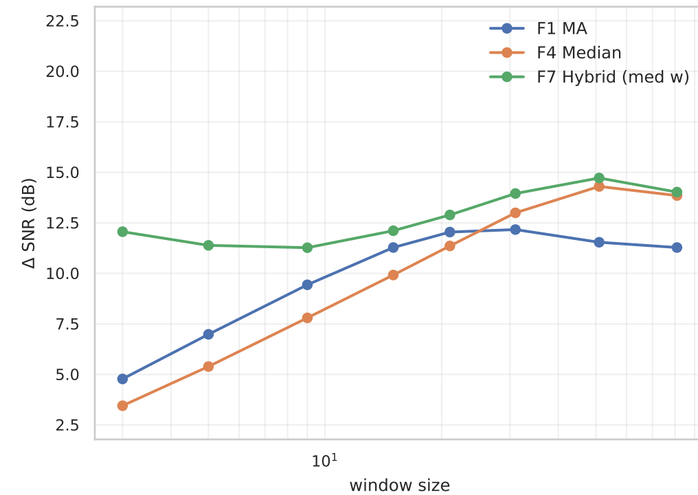
N1 Gauss
