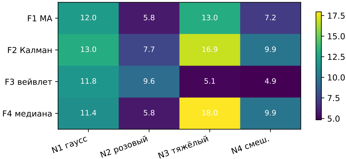
Прирост SNR после фильтрации, дБ
