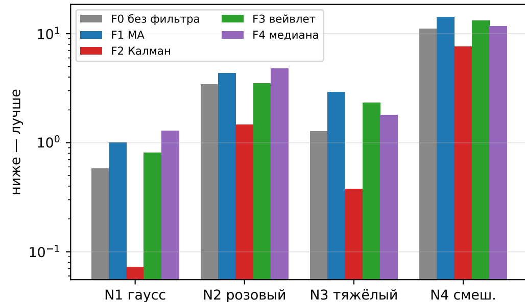
Квадратичная: шумовой пол (медиана \|\nabla f\|^2 )
