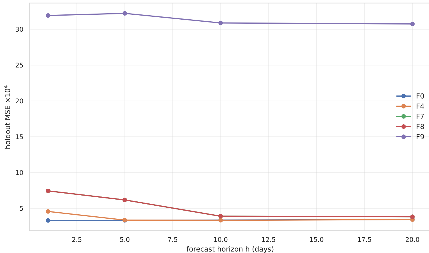
Влияние фильтра на multi-step ahead прогноз
