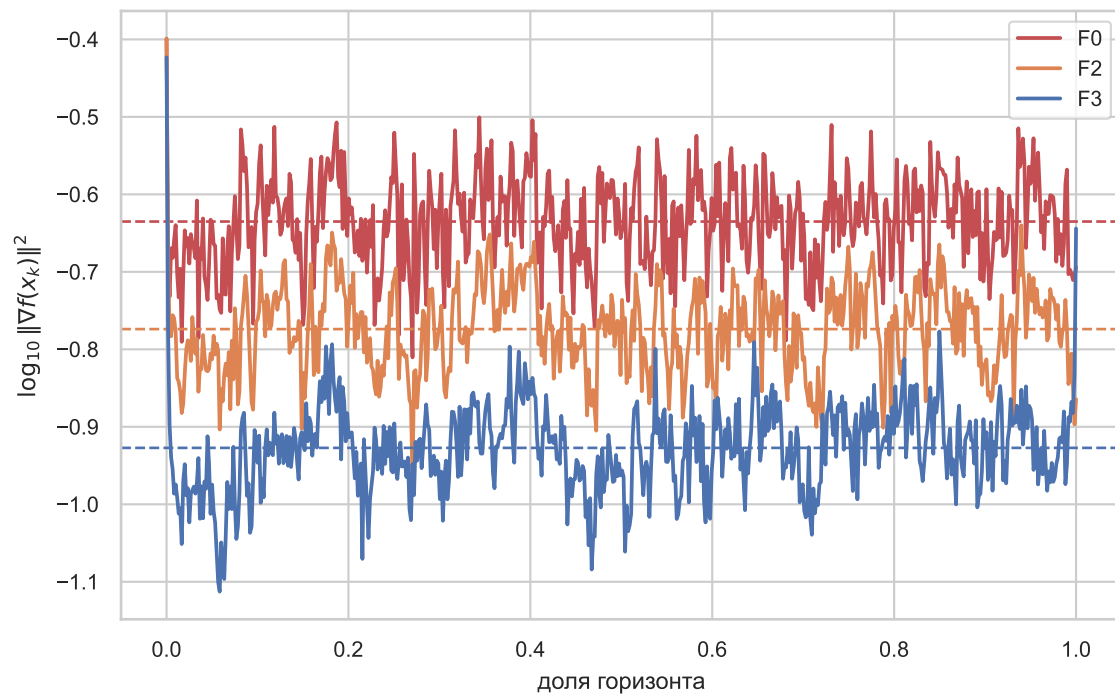
(а) лог-кривые; пунктир — среднее (= AUC)
