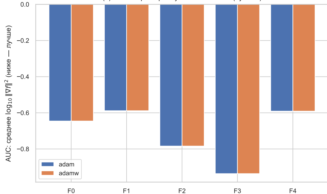
(б) AUC по фильтрам: у F3 наименьшая (лучшая)
