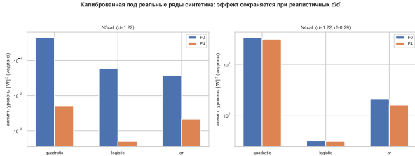
Рис. 5: Синтетика, откалиброванная под реальные \hat{\alpha} и \hat{d} . При тяжёлохвостовом N3cal разрыв F0/F4 сохраняется (91–120×). При смешанном N4cal разрыва нет.
