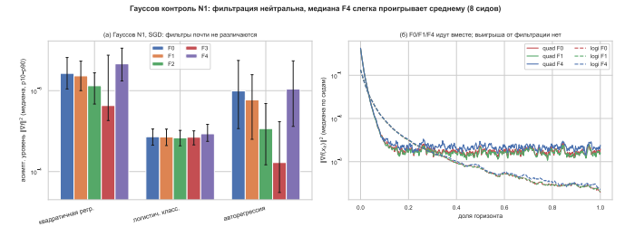
Рис. 2: Гауссов шум N1, SGD, 8 сидов. Слева — асимптотические уровни \|\nabla f\|^2 для F0–F4 почти совпадают по задачам (лог-шкала, полоса p10–p90). Справа — медианные кривые \|\nabla f\|^2 : F0, F1 и F4 идут вместе, выигрыша от фильтрации нет.
