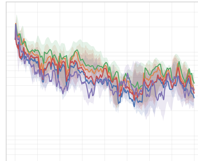
N4 Смешанный
