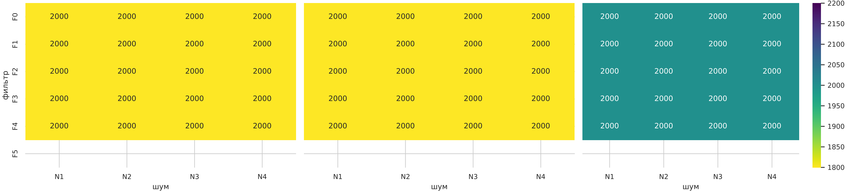
SGD
