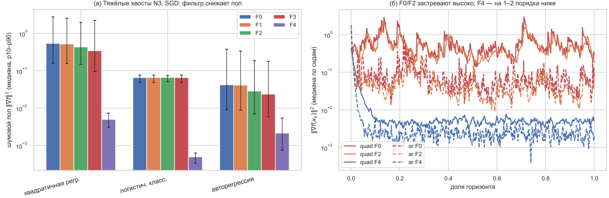
Рис. 1. N_3 , SGD, 8 сидов. (а) асимптотический уровень \|\nabla f\|^2 для F_0 – F_4 , лог-шкала, p_{10} – p_{90} ; (б) медиана \|\nabla f\|^2 : F_0/F_2 застревают, F_4 падает на 1–2 порядка. Линейные и вейвлет-фильтры идут вдоль F_0 (Утверждение 1).
