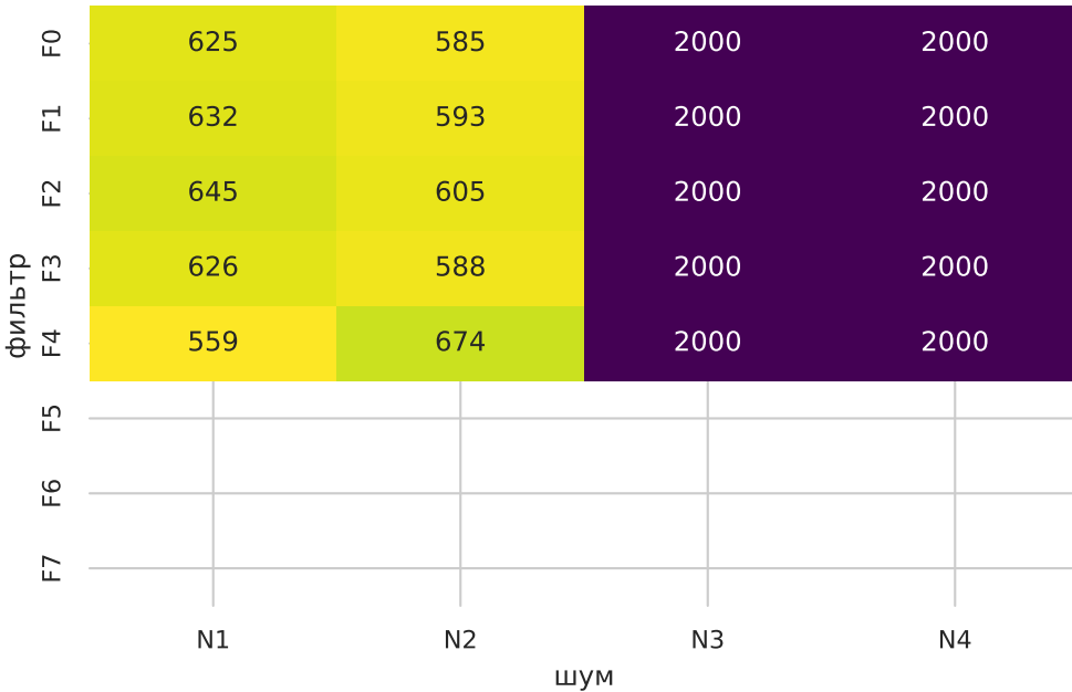
SGD
