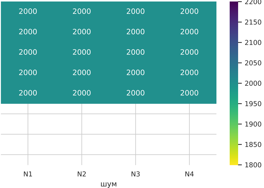
AdamW
