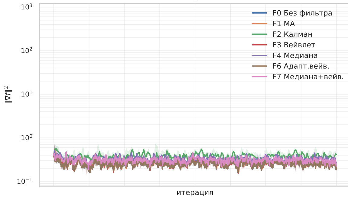
N3 α-устойчивый
