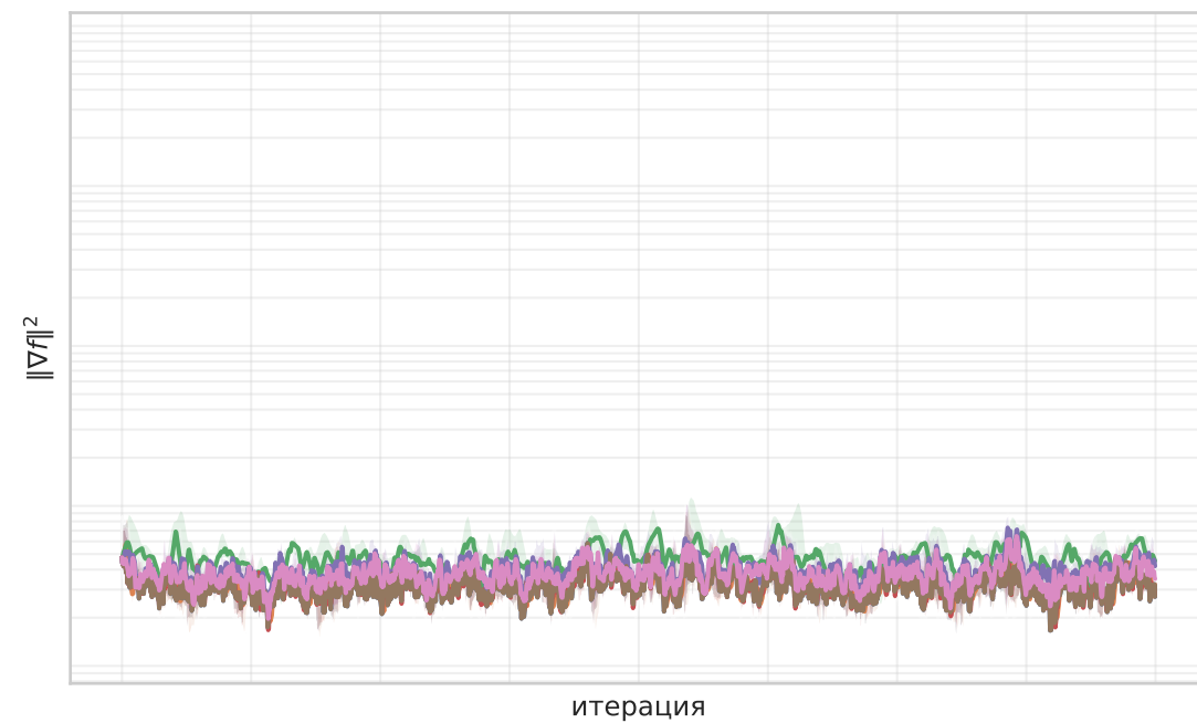
N4 Смешанный
