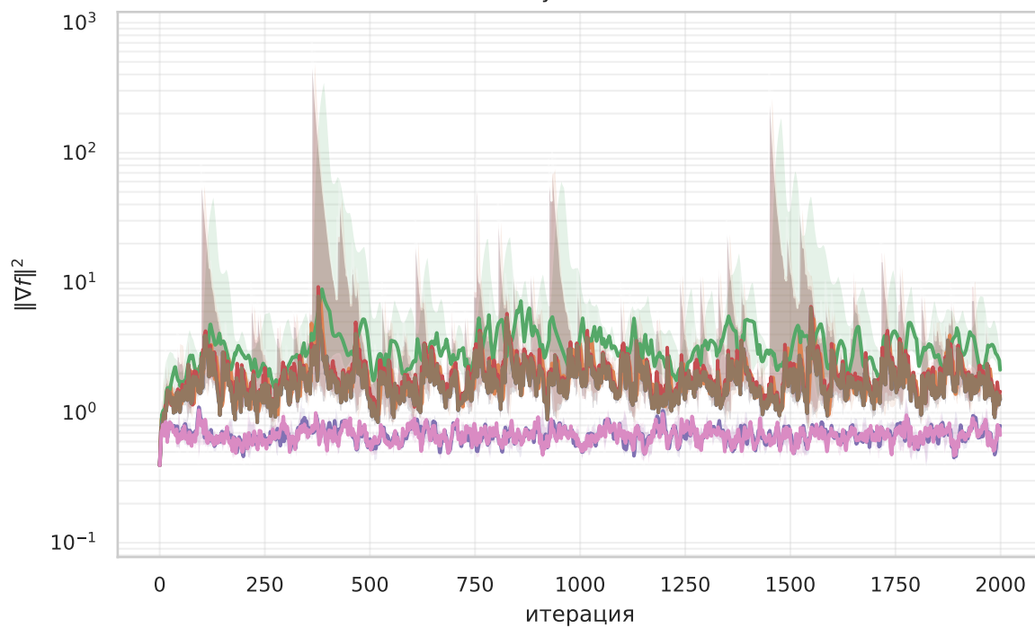
N3 α-устойчивый
