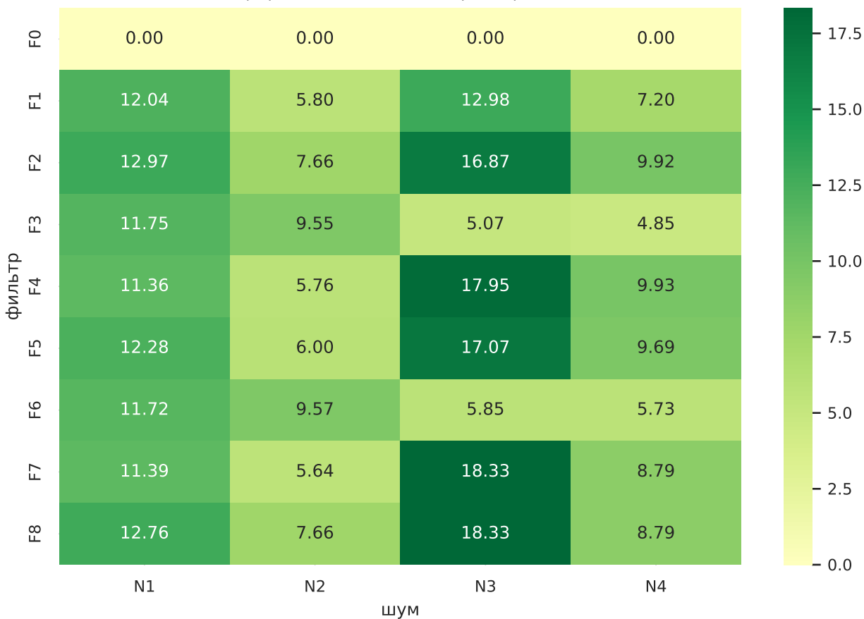
Прирост SNR (дБ) после фильтрации
