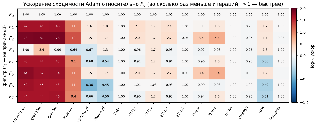
Рис. 2. Полная карта блока D: все фильтры F_0 – F_7 на всех 17 доменах (Adam, регрессия AR(5), 4 сида). Цвет — ускорение сходимости относительно F_0 (во сколько раз меньше итераций до 100\times -снижения \|\nabla f\|^2 ; > 1 — быстрее). Выигрыш сосредоточен на тяжёлохвостовых доходностях (левый блок): линейный Калман F_2 и каскад F_5 дают 44–80×; на светлохвостовых/гладких рядах (FRED, ETT, NOAA, sunspots) все фильтры \approx 1\times . F_3 не причинный (использует будущее) и в правило не входит.
