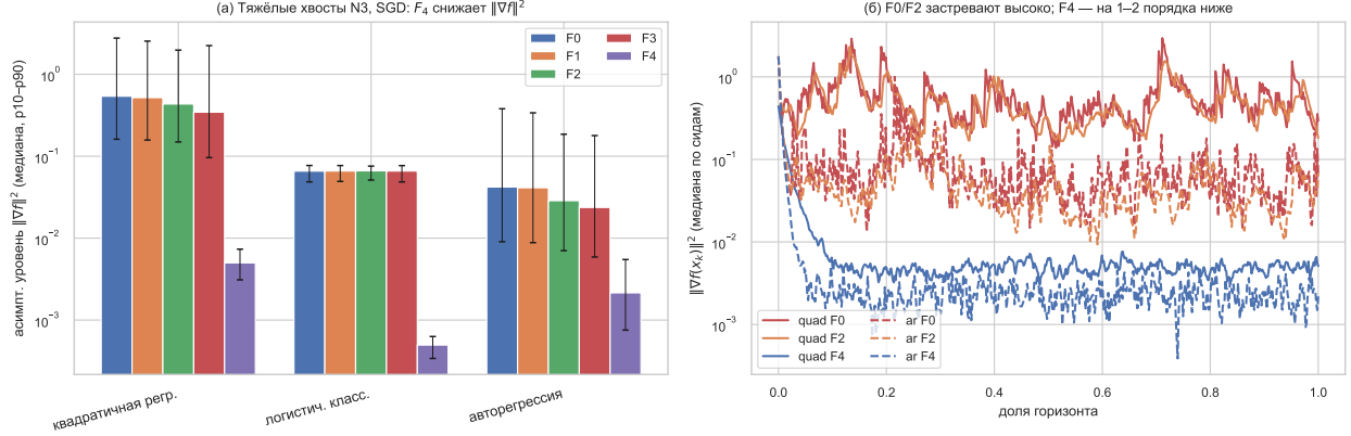
Рис. 1. N_3 , SGD, 8 сидов. (а) асимптотический уровень \|\nabla f\|^2 для F_0 – F_4 , лог-шкала, p_{10} – p_{90} ; (б) медиана \|\nabla f\|^2 : F_0/F_2 застревают высоко; F_4 падает на 1–2 порядка. Линейные и вейвлет-фильтры идут вдоль F_0 (Утверждение 1).
