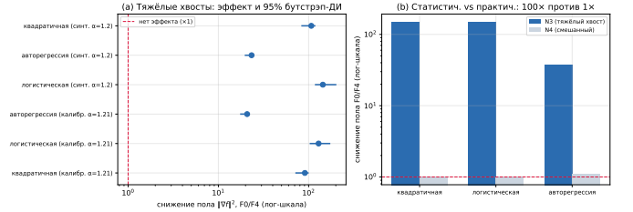
Рис. 5: Слева — лесовидная диаграмма снижения асимптотического уровня F0/F4 при тяжёлых хвостах с 95%-ми бутстрэп-интервалами: для всех задач — и на синтетике ( \alpha = 1.2 ), и на калиброванном под реальные данные шуме ( \alpha = 1.21 ) — интервал целиком правее линии «нет эффекта» ( \times 1 ). Справа — контраст статистической и практической значимости: на N3 фильтр снижает пол в \sim 100 раз, на смешанном N4 — лишь в \sim 1.1 , у самой границы \times 1 (лог-шкала).
