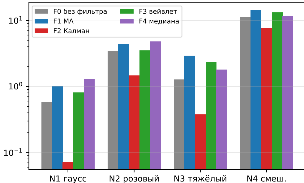
Квадратичная: шумовой пол (медиана \|\nabla f\|^2 )
