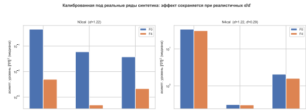
Рис. 4: Синтетика, откалиброванная под реальные \hat{\alpha} и \hat{d} . При тяжёлохвостовом N3cal разрыв F0/F4 сохраняется (91–120×). При смешанном N4cal разрыва нет.
