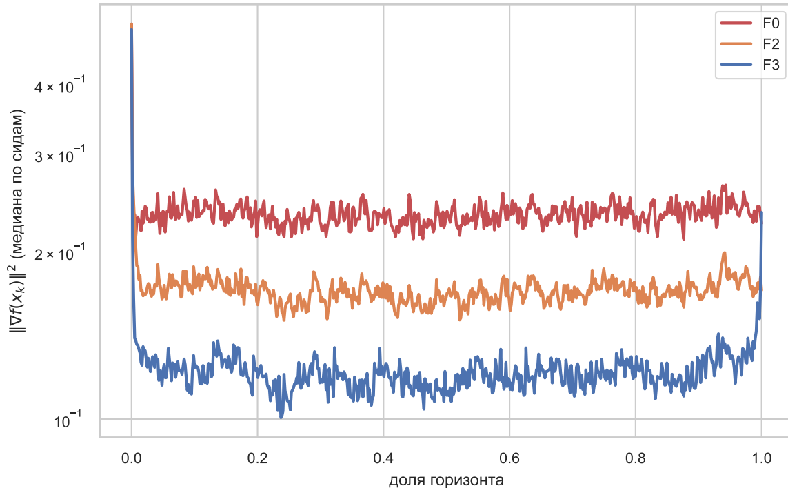
(а) N2, квадратичная, Adam: F3 уходит вниз раньше
