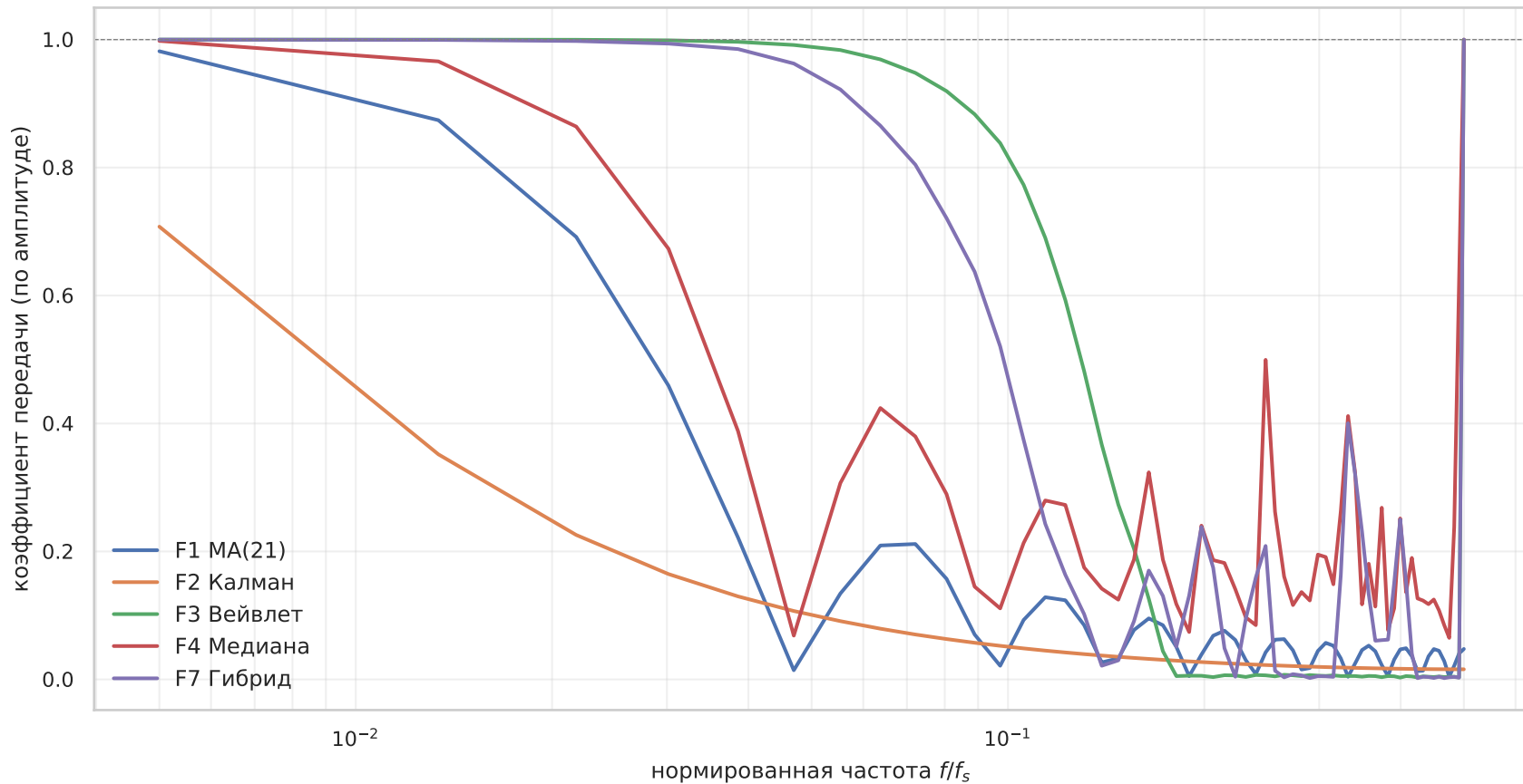
Эмпирический амплитудный отклик фильтров на синусоиду
