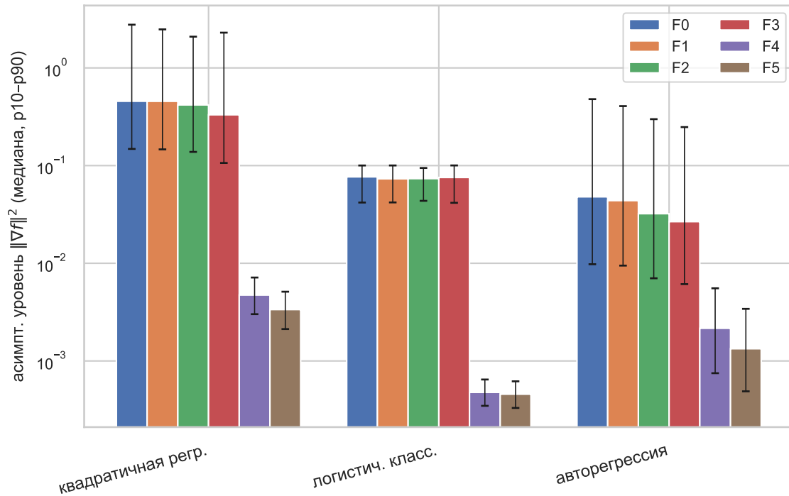
(а) Тяжёлые хвосты N3, SGD: F_4 снижает \|\nabla f\|^2
