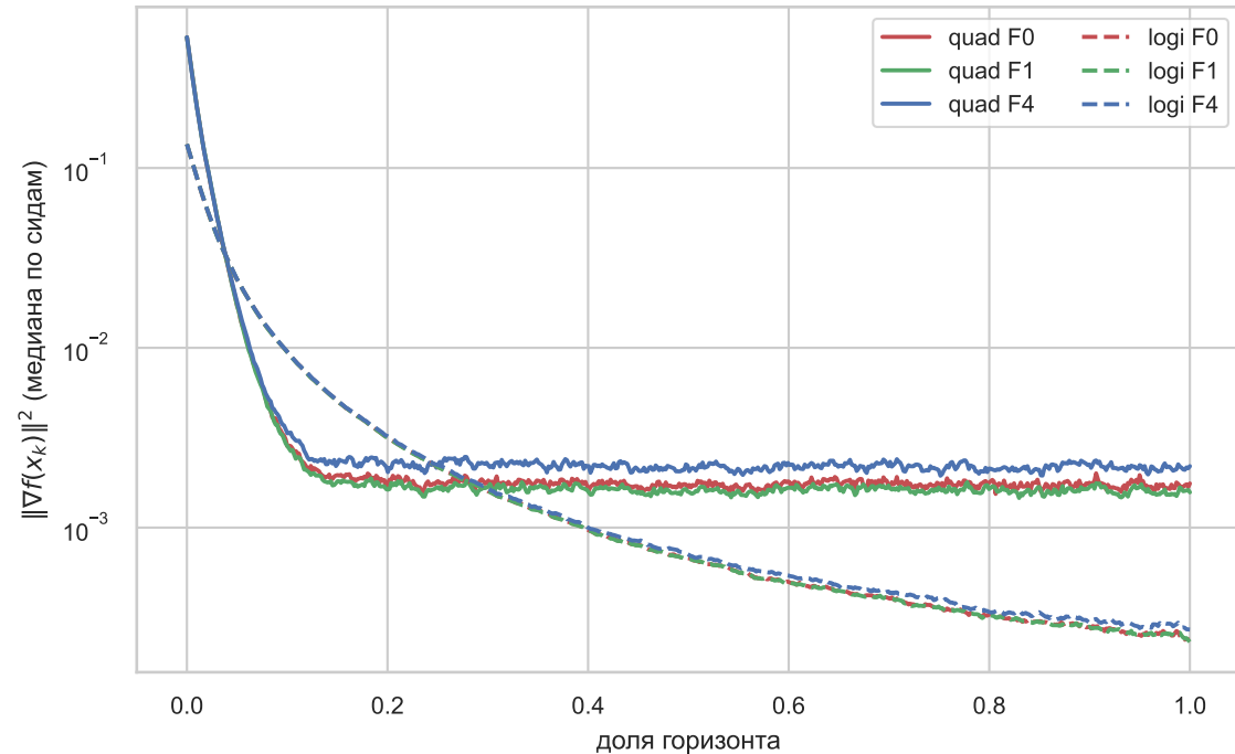
(б) F0/F1/F4 идут вместе; выигрыша от фильтрации нет
