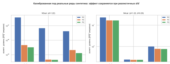
Рис. 6: Синтетика, откалиброванная под реальные \hat{\alpha} и \hat{d} . При тяжёлохвостовом N3cal разрыв F0/F4 сохраняется (91–129×). При смешанном N4cal разрыва нет.
