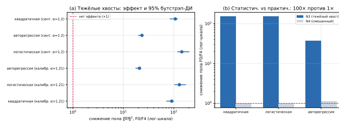
Рис. 5: Слева — лесовидная диаграмма снижения асимптотического уровня F0/F4 при тяжёлых хвостах с 95%-ми бутстрап-интервалами: для всех задач — и на синтетике ( \alpha = 1.2 ), и на калиброванном под реальные данные шуме ( \alpha = 1.21 ) — интервал целиком правее линии «нет эффекта» ( \times 1 ). Справа — контраст статистической и практической значимости: на N3 фильтр снижает пол в \sim 100 раз, на смешанном N4 — лишь в \sim 1.1 , у самой границы \times 1 (лог-шкала).
