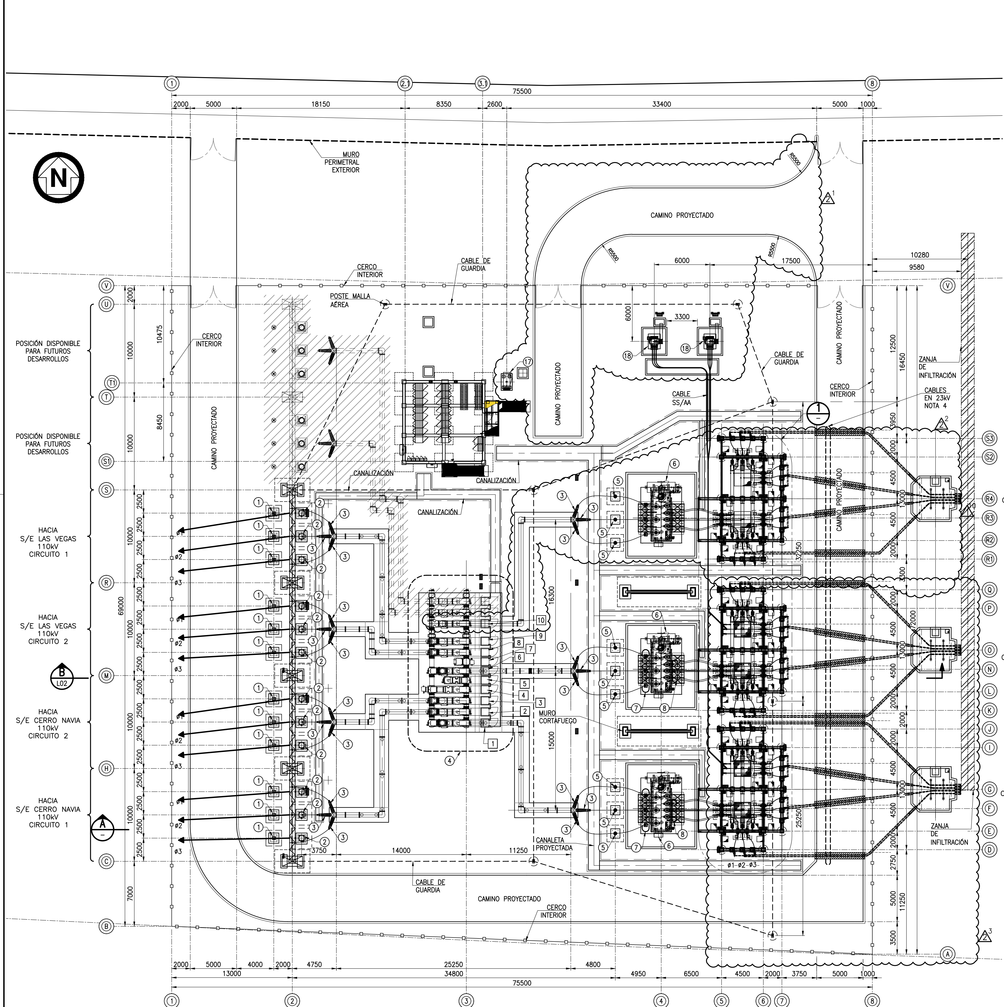
DISPOSICIÓN DE EQUIPOS (PLANTA) - SE SECCIONADORA COLINA 110/23 kV
