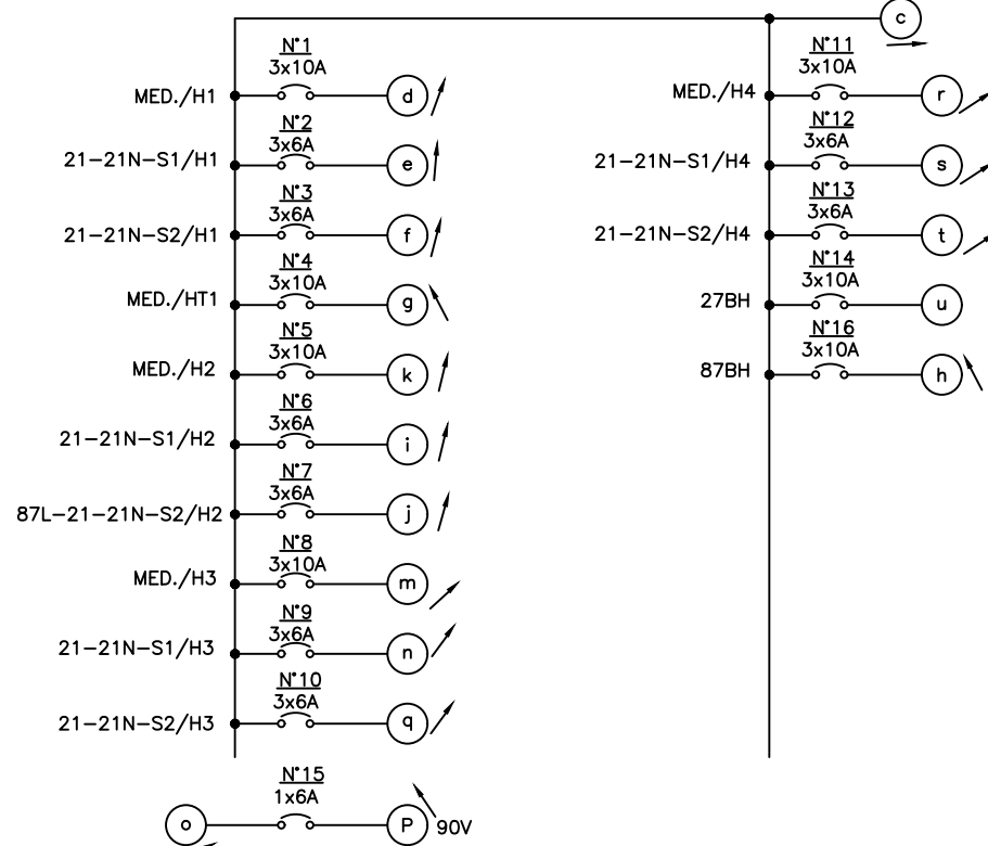
DISTRIBUCION POTENCIALES BARRA 110kV
