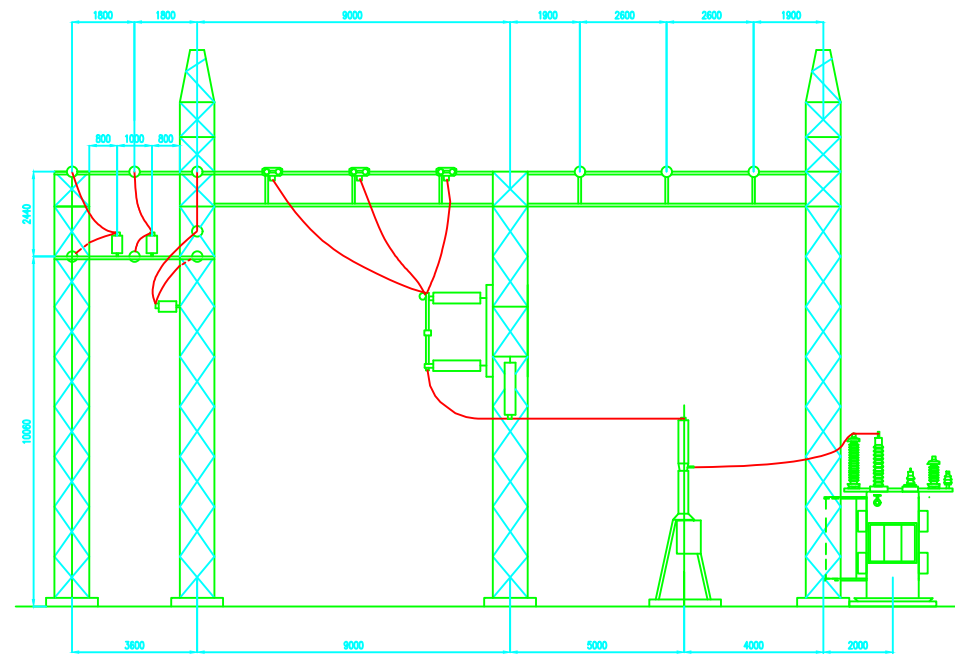
CORTE A ESCALA: 1:100
