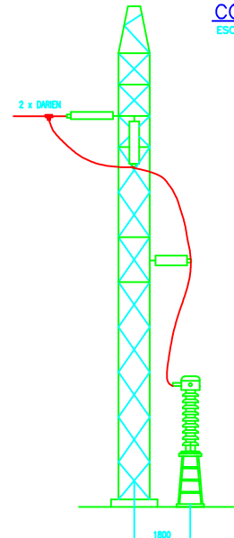
CORTE K ESCALA: 1:100
