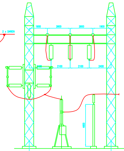
CORTE M ESCALA: 1:100
