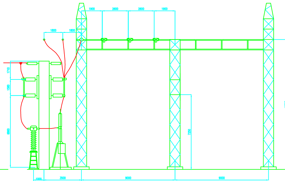
CORTE E ESCALA: 1:100
