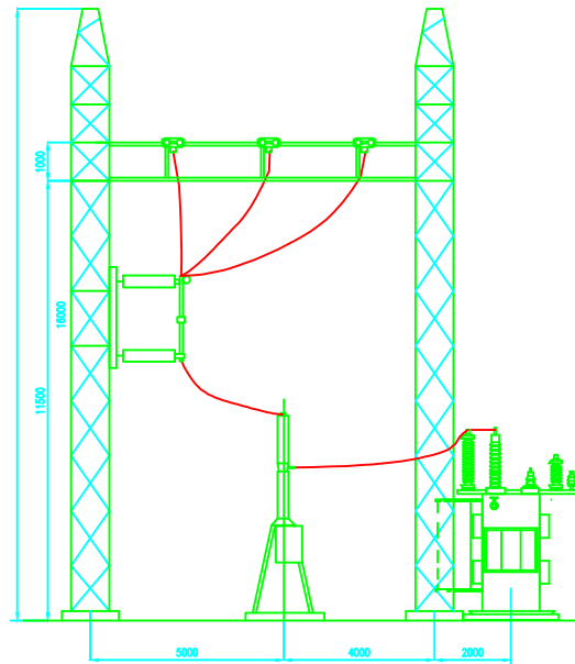
CORTE C ESCALA: 1:100
