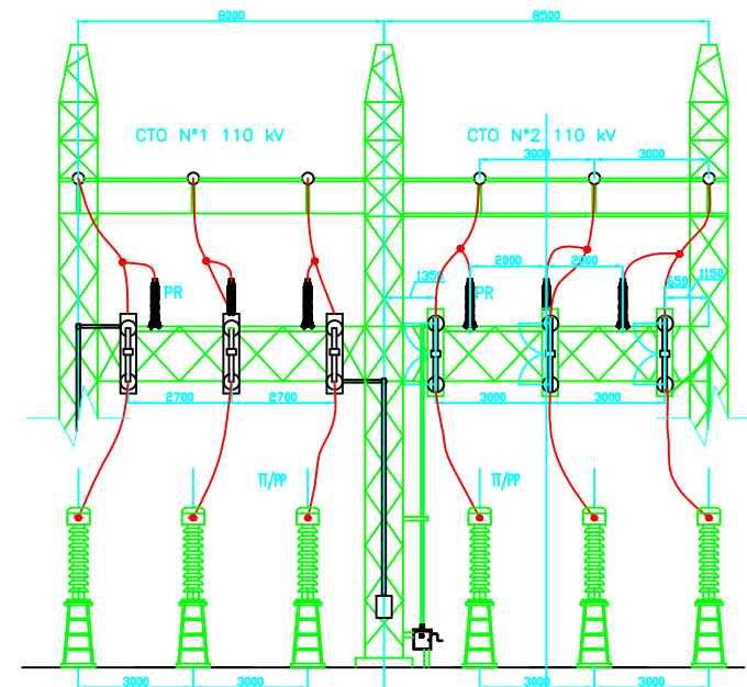
CORTE H ESCALA: 1:100
