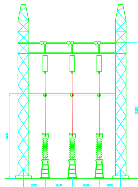
CORTE G ESCALA: 1:100
