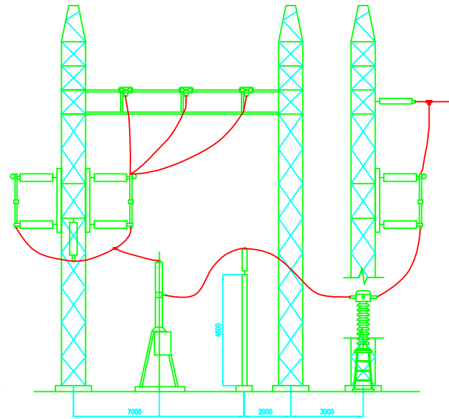
CORTE F ESCALA: 1:100
