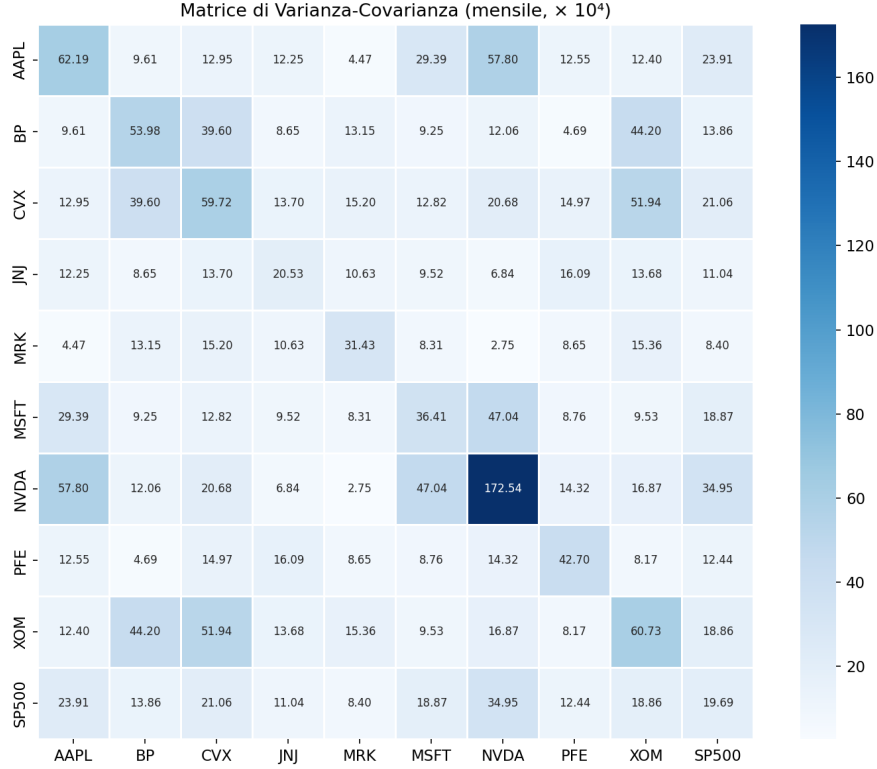
Figura 1: Matrice di varianza-covarianza mensile (valori \times 10^{-4} ). NVDA presenta la varianza più elevata; le covarianze Tech-Energy sono più basse di quelle intra-Tech.
