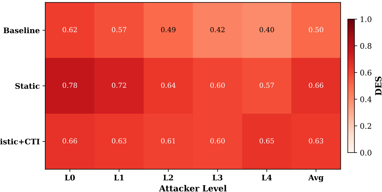
DES Heatmap
