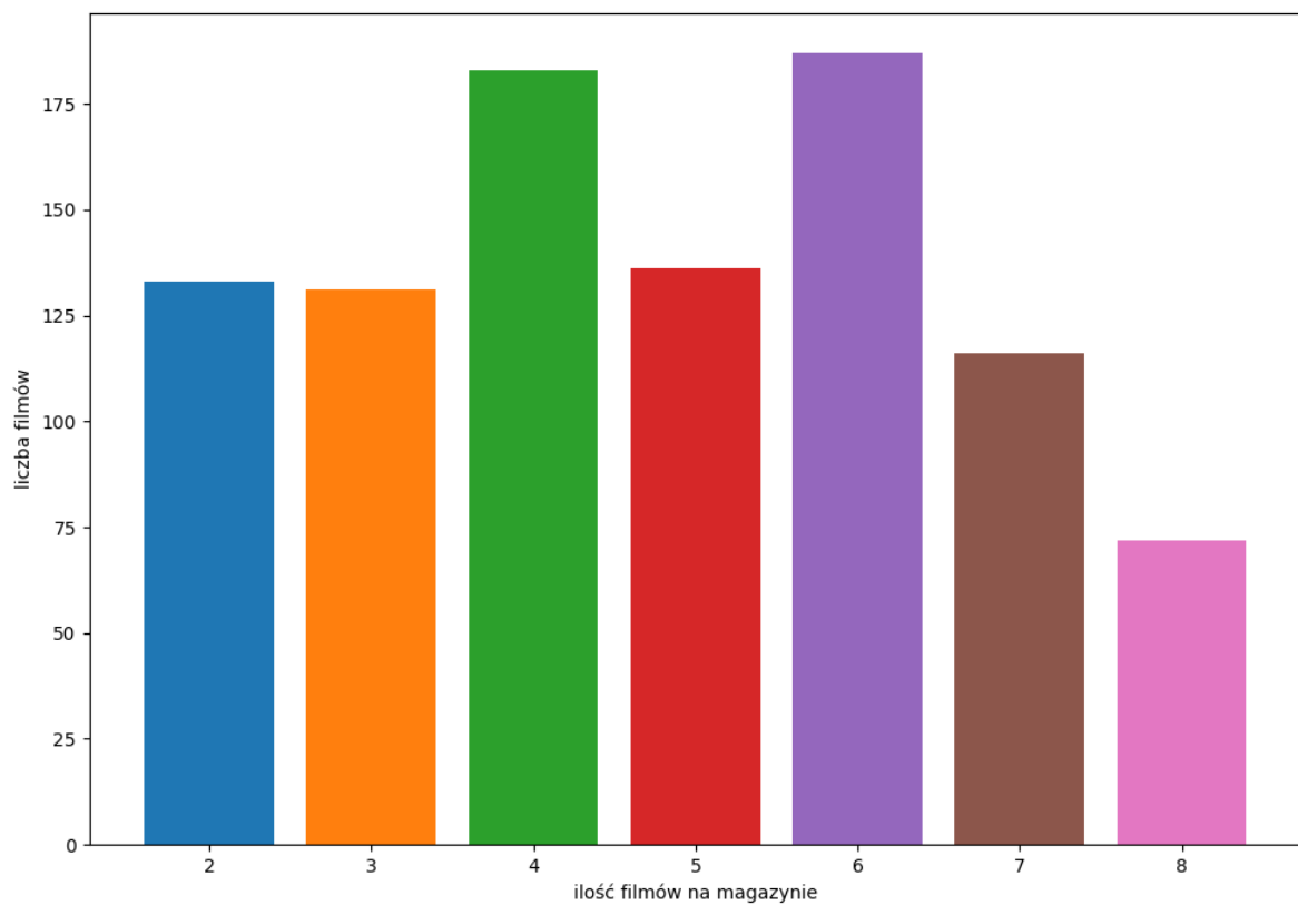
Rysunek 5: Stan magazynowy
