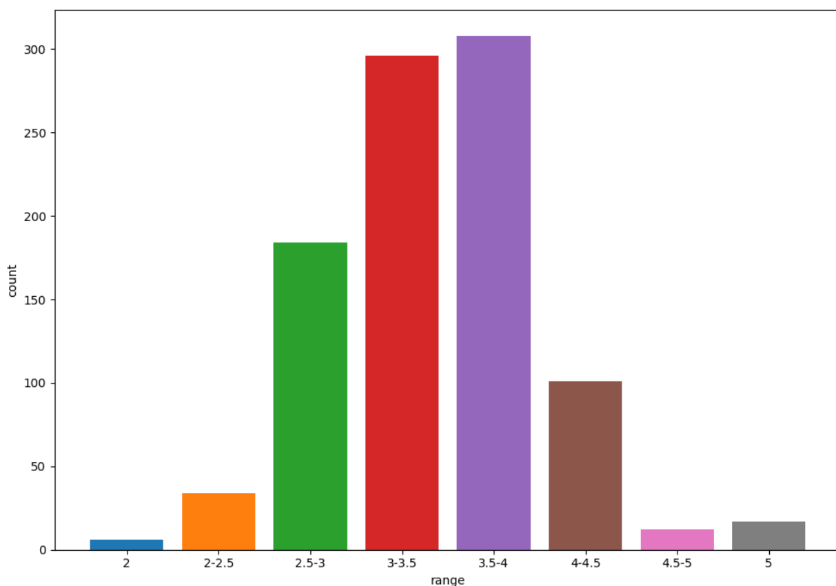
Rysunek 6: Liczba wypożyczeń jednej kopii
