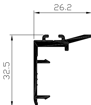
כנף הזזה - שולב מס' פרופיל : 06106 משקל : 333 גרם/מטר היקף כללי : 151 מ"מ
