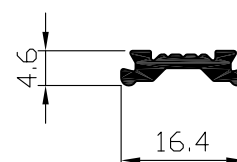
כנף ציר - מוט מזביל מס' פרופיל : 06148 משקל : 114 גרם/מטר היקף כללי : 48 מ"מ
