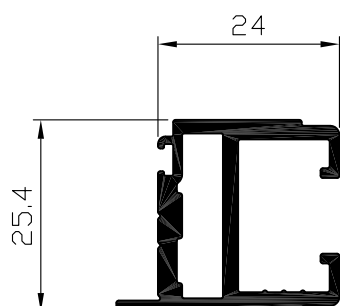
כנף ציר - זיגוג 4 ÷ 6 מ"מ מס' פרופיל : 06087 משקל : 593 גרם/מטר היקף כללי : 220 מ"מ היקף חיצוני : 165 מ"מ
