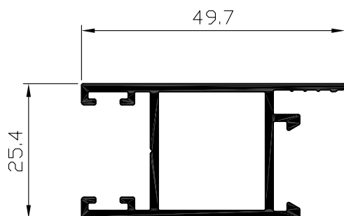
כנף הזזה - צד מס' פרופיל : 06089 משקל : 621 גרם/מטר היקף כללי : 314 מ"מ היקף חיצוני : 229 מ"מ
