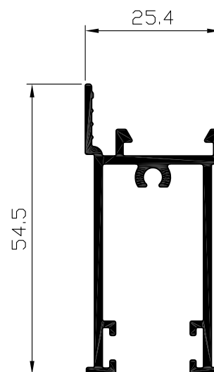
כנף הזזה - עליון/תחתון מס' פרופיל : 06083 משקל : 622 גרם/מטר היקף כללי : 311 מ"מ
