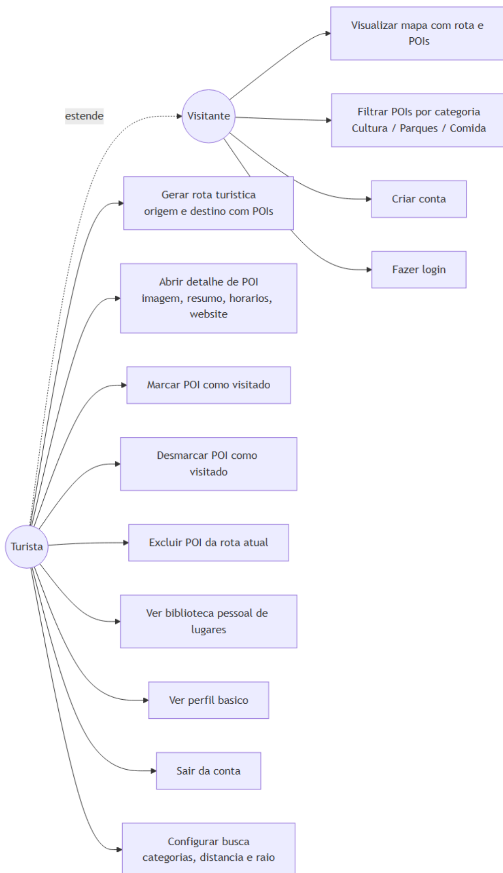
Figura 5: Diagrama de casos de uso – MVP
