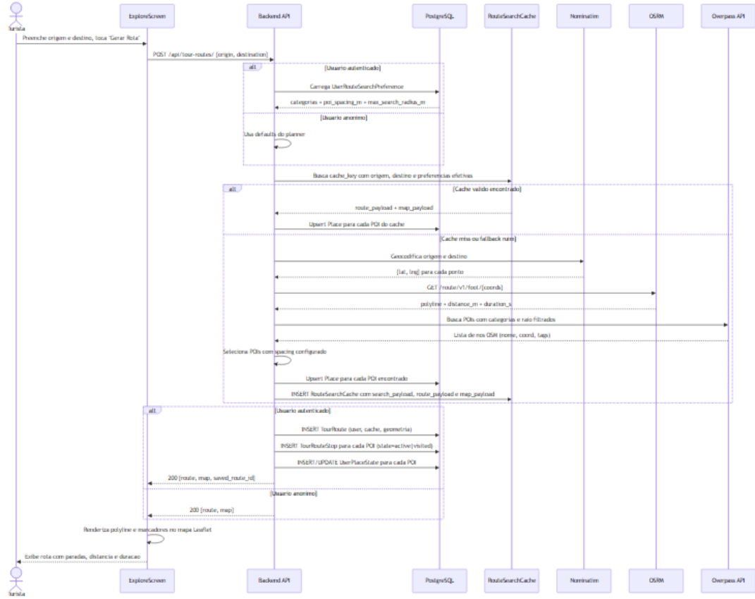
Figura 6: Diagrama de sequência – Gerar Rota
