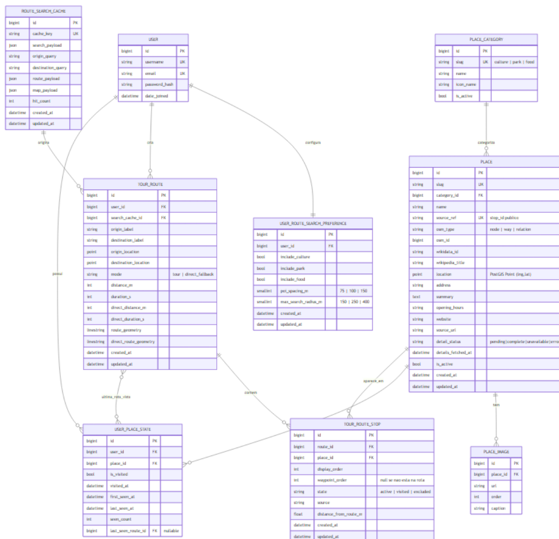
Figura 3: Diagrama ER do Explora+ – MVP entregue
