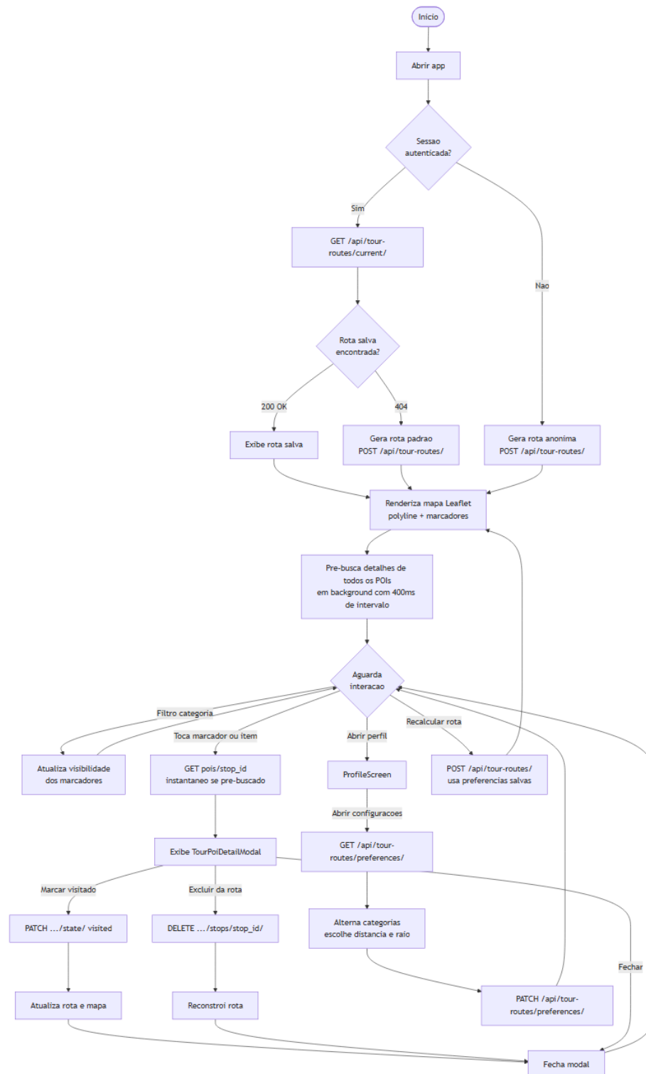
Figura 9: Diagrama de atividade – Fluxo da ExploreScreen
