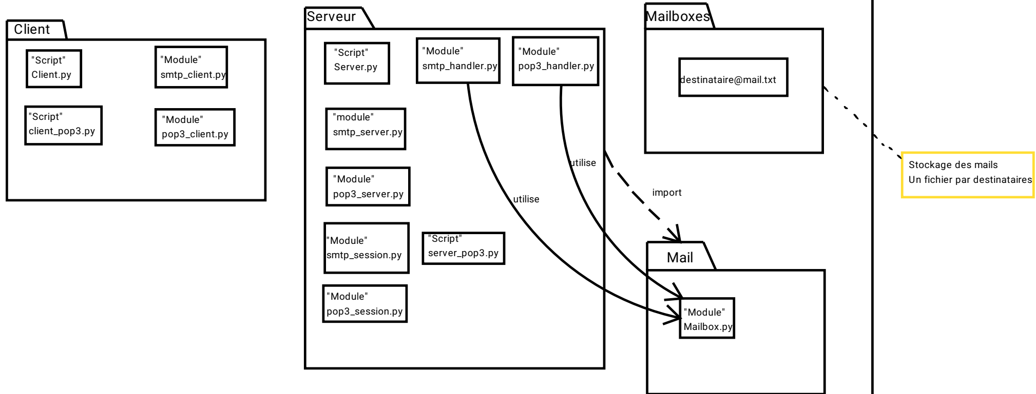
Diagramme de package - Projet SMTP
