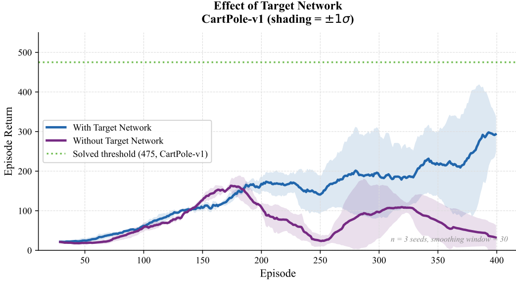
图 3: 目标网络的消融实验 (CartPole-v1, 3 个随机种子, 阴影为 \pm 1\sigma )。无目标网络时, 训练曲线更不稳定, 种子间方差更高。
