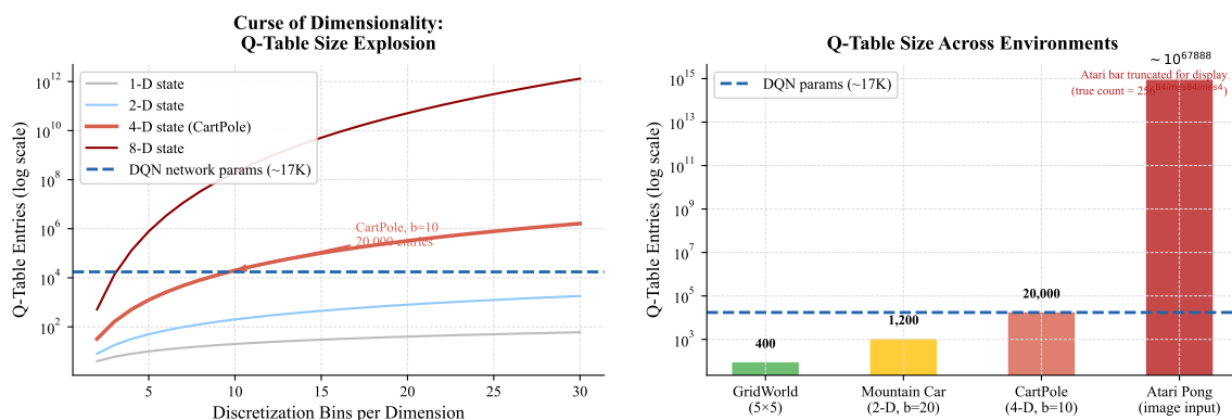
图 1: 维度灾难: Q 表大小随状态维度和离散化精度指数爆炸, 远超一个小型神经网络的参数量。
