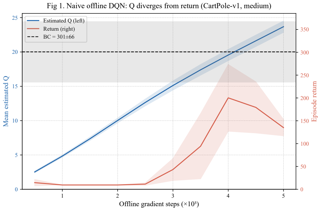
图 1: 朴素离线 DQN 的外推误差塌缩 (CartPole-v1, medium 数据集, 3 个随机种子, 阴影为 \pm 1\sigma )。同一张图里：蓝色曲线（左轴）是 Q 网络对数据状态的最大 Q 估计——它不再跟踪策略的真实价值；红色曲线（右轴）是贪心策略的真实回报，短暂改善后回落，且始终远低于行为克隆（BC）这条「及格线」（BC 约 300，见图 2 的灰色区间）。Q 估计与真实回报脱钩——正是外推误差进入自举目标后的表现。
