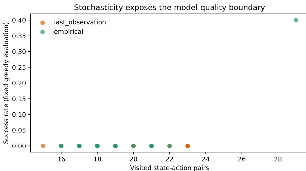
图 3: 随机 FrozenLake-v1 中 last-observation 与 empirical 模型的覆盖—成功率诊断; 每个点对应一个 seed, 成功率来自固定、无探索的贪心评估。该图比较模型表示方式, 不把相关性夸大为因果结论。
