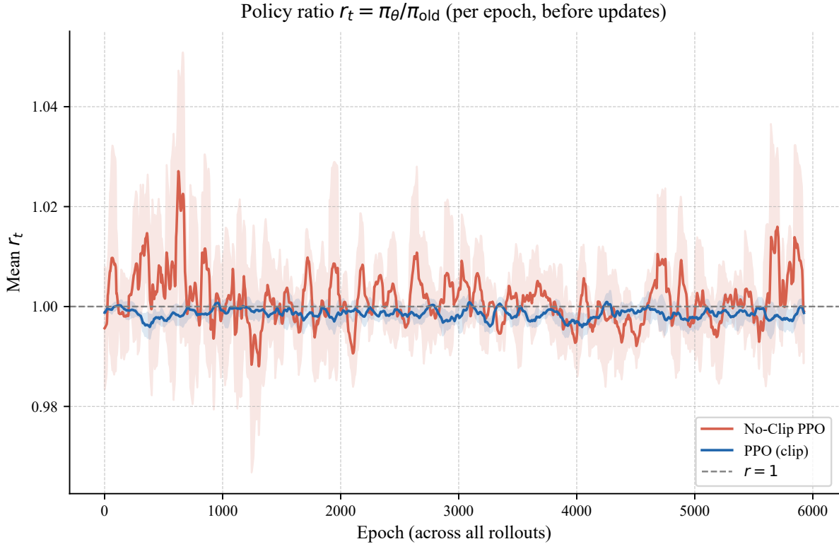
图 3: 每个 epoch 开始前、以全批数据测量的均值策略比值 r_t (5 seeds, 均值 \pm 标准差)。无 Clip (红) 偏离更大, 早期可达 \sim 1.017 ; PPO-Clip (蓝) 始终贴近 1。均值之外, 个别 transition 的 r_t 可远超 1.2 的 clip 边界, 正是这些尾部被 clip 截断, 防止了错误梯度的累积。
