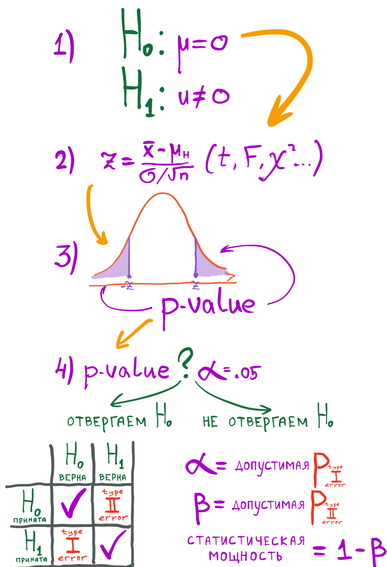
Рисунок 17.6: Схема этапов тестирования значимости нулевой гипотезы
