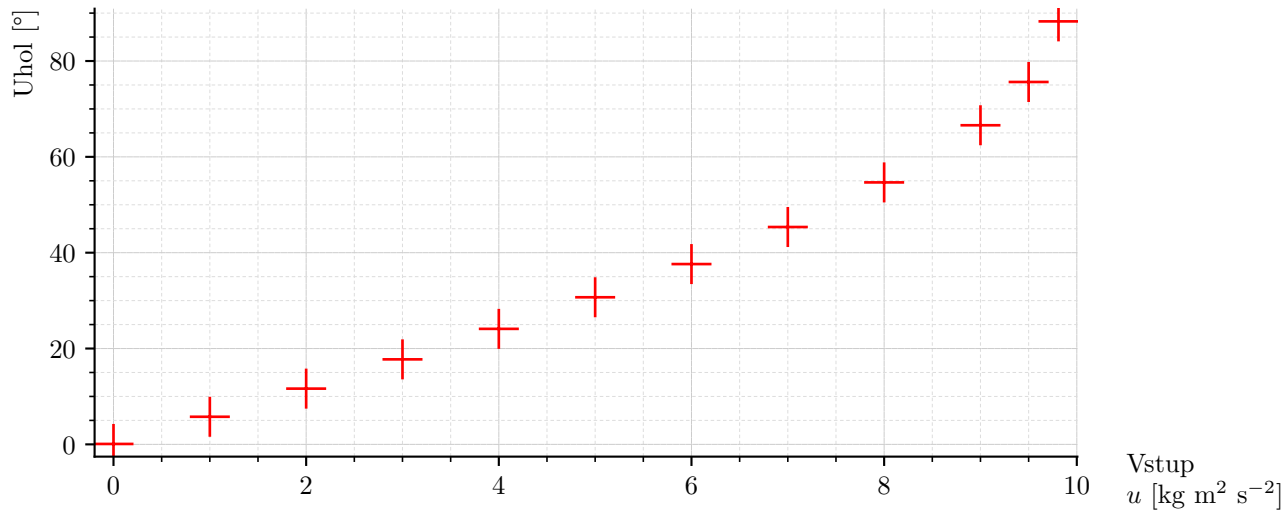
Prevodová charakteristika
