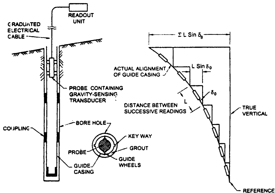
FIG. 1 PROBE INCLINOMETER
