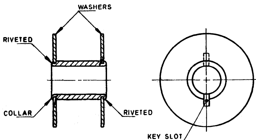
FIG. 1 NOMENCLATURE FOR BOBBINS
