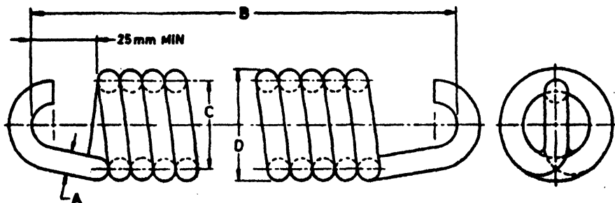
FIG. 2 SPRING
