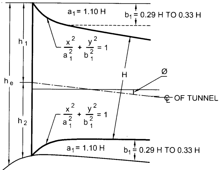
8A ELEVATION
